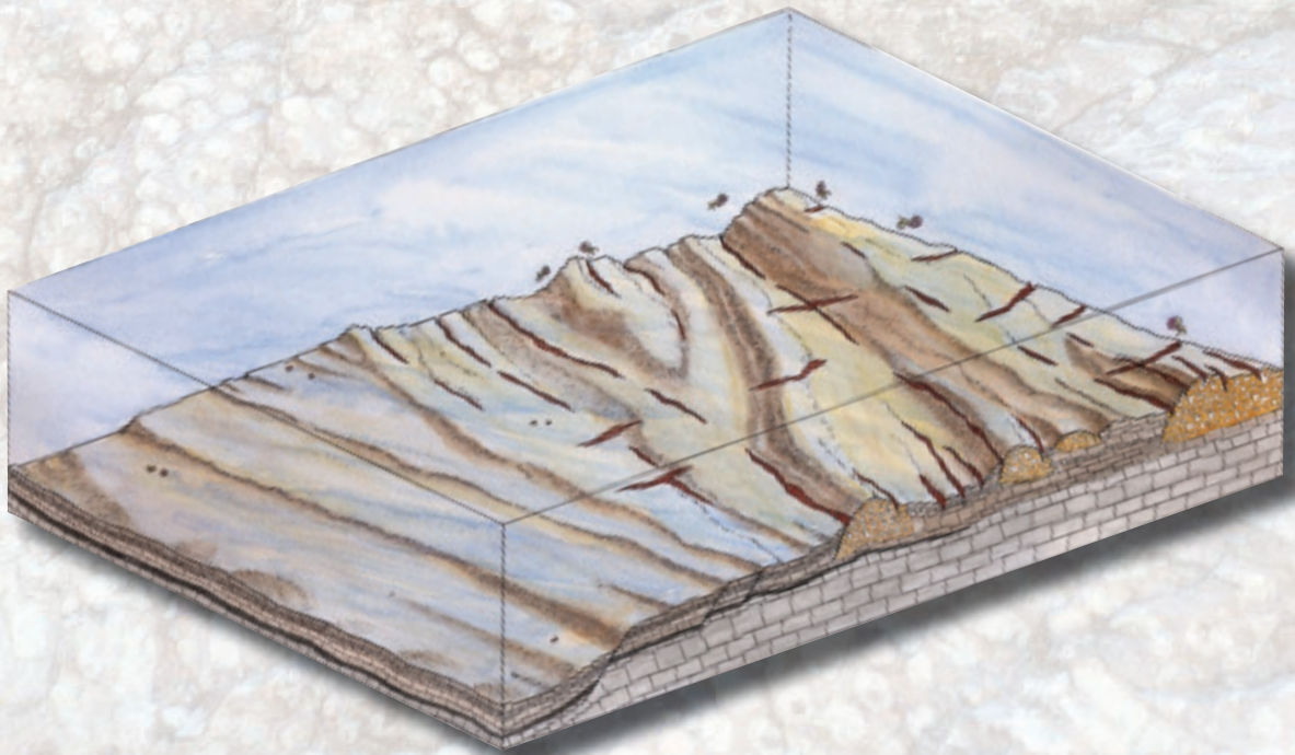
Darstellung des Ablagerungsraumes der bunten Liaskalke von Adnet; die Ablagerung erfolgte auf Tiefschwellen in einem sich absenkenden Meeresbecken; Karstspalten in den Rhät-Riffkalken wurden mit Eisenoxid-reichem roten Ton verfüllt.
