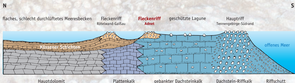
Schematischer Nord-Süd-Schnitt durch den Ablagerungsraum um das Adnetter Fleckenriff während der obersten Trias (nach H. Kretschmer, 1986)
