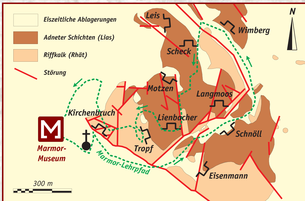
Geologische Kartenskizze des Steinbruch-Gebietes von Adnet (verändert nach B. Plöching, 1990); charakteristisch ist die Zerstückelung des Kalkstockes in eine Vielzahl von Bruchschollen
