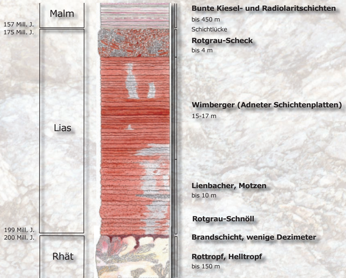
Schematisches Säulenprofil der Schichtenfolge von Adnet
